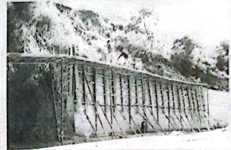
En la vereda Media Luna poco a poco avanza el gigante muro de contención que se construye en la margen izquierda bajando sobre la vía a Santa Elena. Varios operarios descargan los coches con el concreto hasta darle la altura definida en los diseños. Este muro de contención dará estabilización al talud que en el pasado invió el sitio con múltiples derrumbes obstaculizando el paso del tránsito vehicular. (Foto León Darío Posada)
